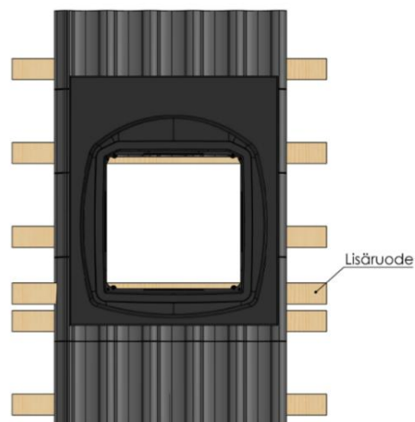
Kuva 2. Ruoteet
