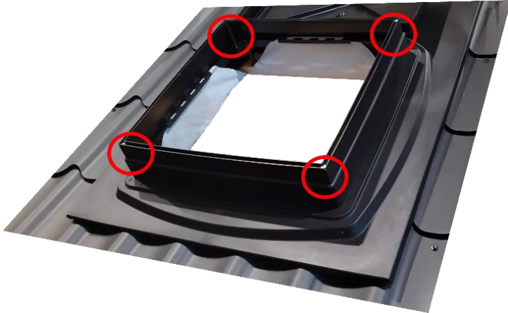
Kuva 8. Ruuvien paikat
